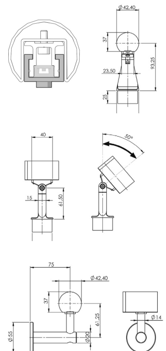
Voorbeeld afmetingen ILLUNOX® type 42,4: dwars- doorsnede, balusteradapter en leuningdrager
